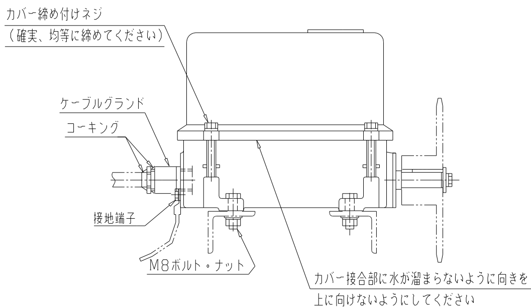
図 3-1 据付け例
