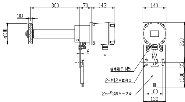
LSA-01-1 外形図
